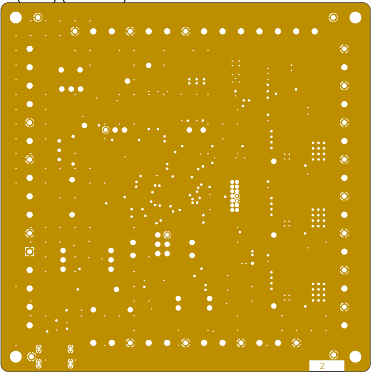
L2(PWR) (Scale 1:1)
